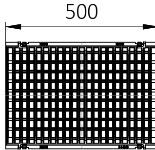
POHLED ZDOLA
