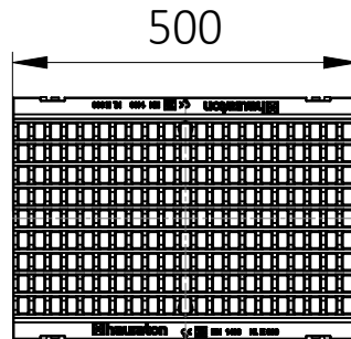
POHLED SHORA
