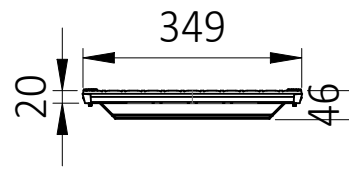
POHLED ZČELA
