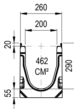
POHLED ZČELA
