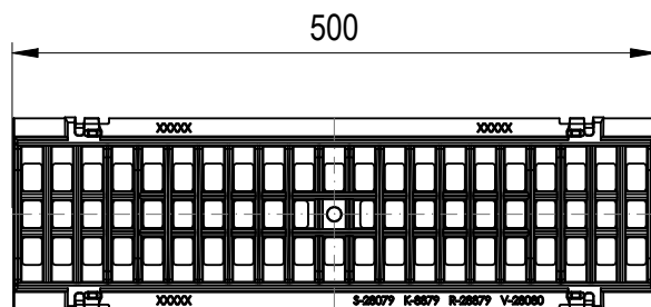
POHLED ZDOLA
