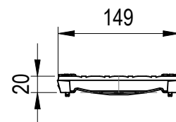
POHLED ZČELA
