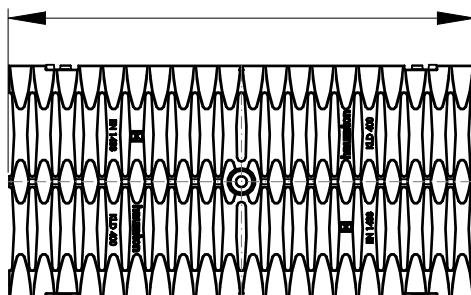
POHLED SHORA
