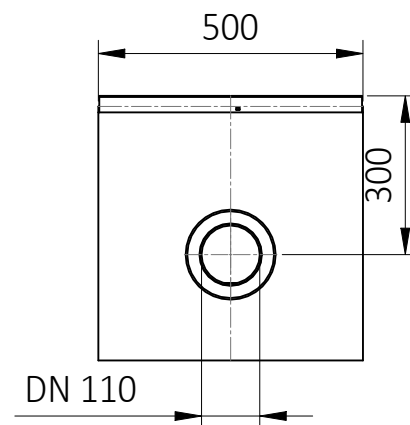
POHLED ZPRAVA
