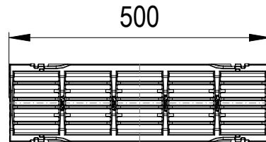
POHLED ZDOLA
