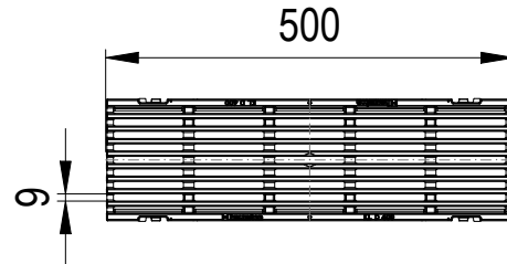
POHLED SHORA
