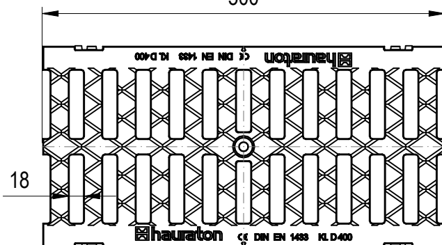
POHLED SHORA
