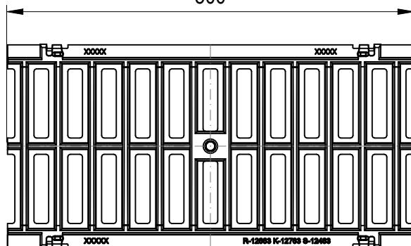
POHLED ZDOLA
