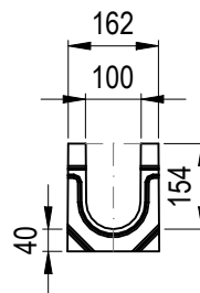
POHLED ZČELA
