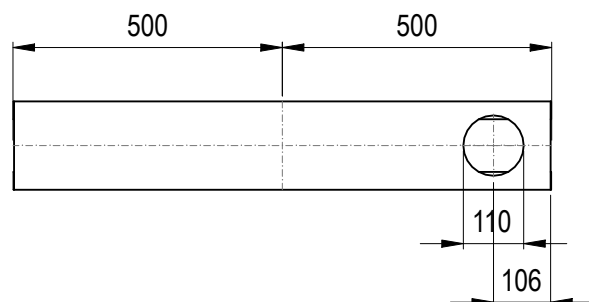
POHLED ZPRAVA (SMĚR TOKU →)
