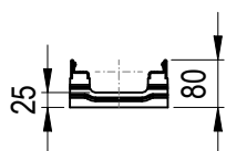
POHLED ZPŘEDU
