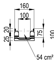
POHLED ZČELA
