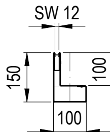
POHLED ZČELA
