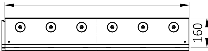
POHLED SHORA
