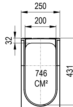
POHLED ZE ZADU
