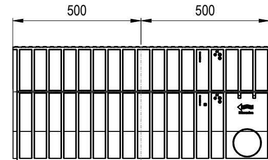
POHLED ZLEVA
