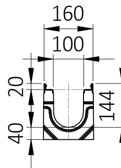
POHLED ZE ZADU
