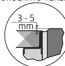
DETAIL ULOŽENÍ U OKOLNÍHO TERÉNU
