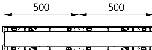
POHLED SHORA
