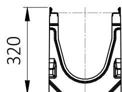
POHLED ZPŘEDU
