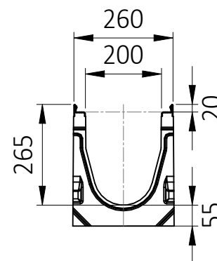
POHLED ODZADU
