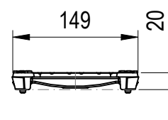
POHLED ZČELA
