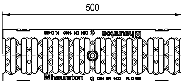
POHLED SHORA
