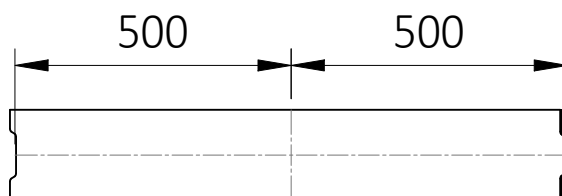
POHLED ZPRAVA (SMĚR TOKU →)
