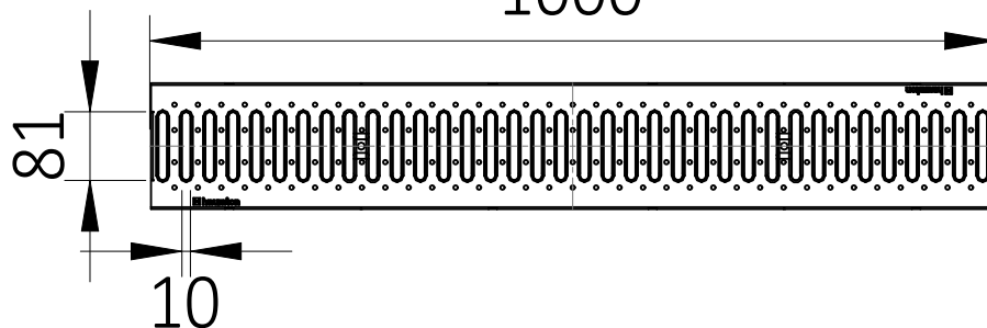
POHLED SHORA
