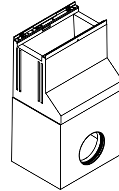
PROSTOROVÉ ZOBRAZENÍ
