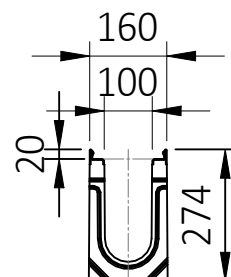
POHLED ODZADU
