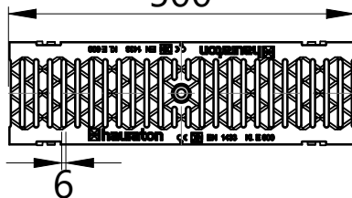
POHLED SHORA
