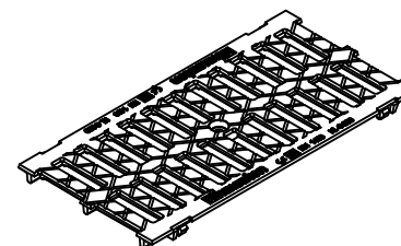
PROSTOROVÉ VYOBRAZENÍ
