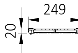
POHLED ZČELA
