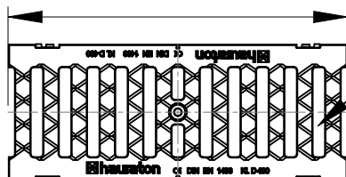
POHLED SHORA 500
