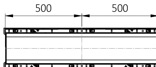
POHLED SHORA
