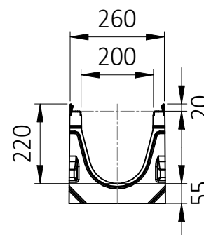
POHLED ZE ZADU
