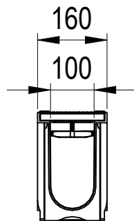
POHLED ZČELA
