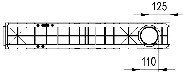
POHLED ZDOLA
