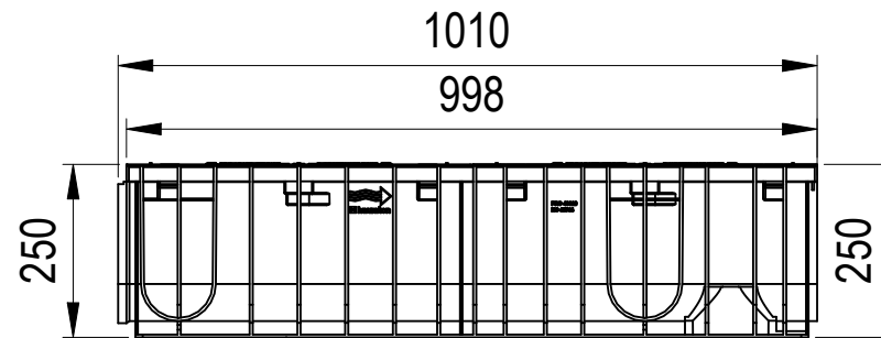
POHLED ZPRAVA
