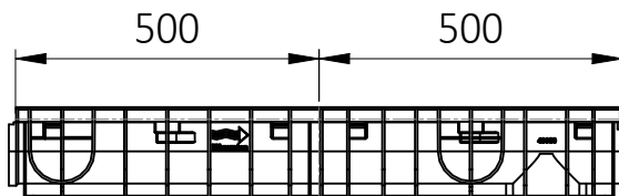
POHLED ZPRAVA (SMĚR TOKU →)
