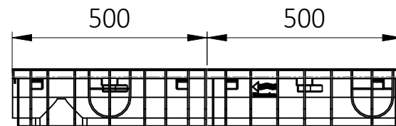
POHLED ZLEVA
