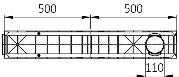
POHLED ZDOLA
