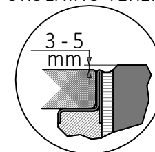
DETAIL ULOŽENÍ U OKOLNÍHO TERÉNU
